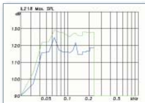
Max. SPL
